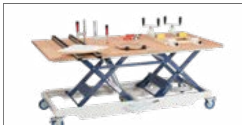
Niveau-Hubtisch Beck HS 300 gross mit Buchen-Lochraster-Arbeitsplatte, mit Zubehör
