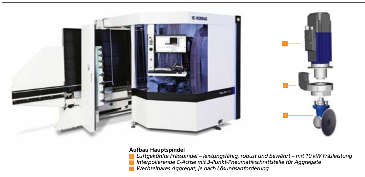
Vertikales CNC-Bearbeitungszentrum HOMAG DRILLTEQ V-310
